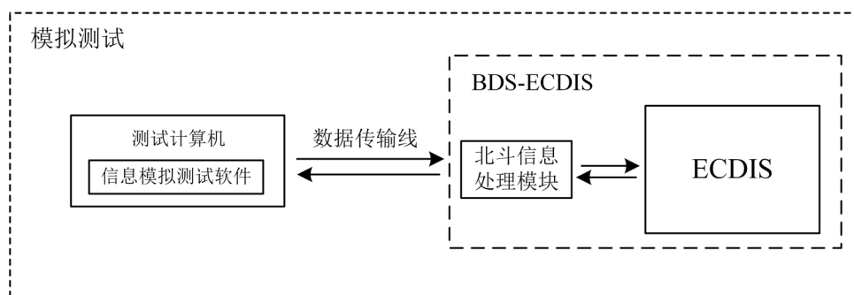
图2 BDS-ECDIS与模拟测试设备连接示意图
