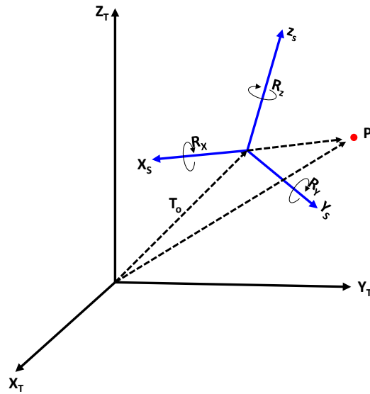
图 2 坐标系三维转换的平移和旋转
