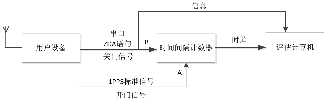
图10 串口输出信号实星环境检定连接框图
